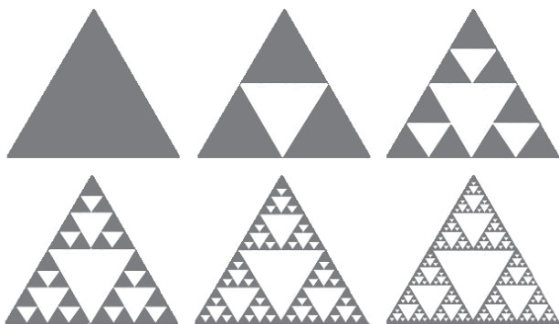
Obrázek č. 65. Fraktál Sierpinského trojúhelník Proces konstrukce fraktálu v trojúhelníku cestou neustálého opakovaní dělení na čtyři různé rovnoramenné trojúhelníky.
