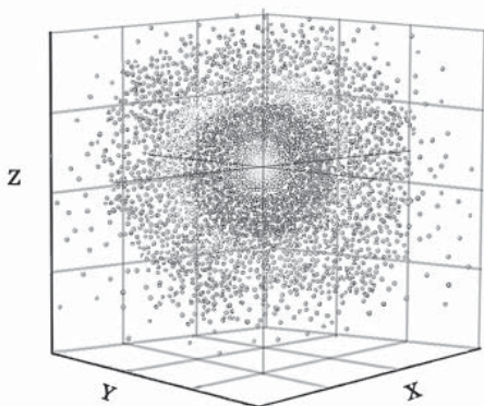
Obrázek č. 2. Elektronový oblak atomu vodíku: část trojrozměrného prostoru okolo atomového jádra, kde se s největší pravděpodobností nachází elektron.
