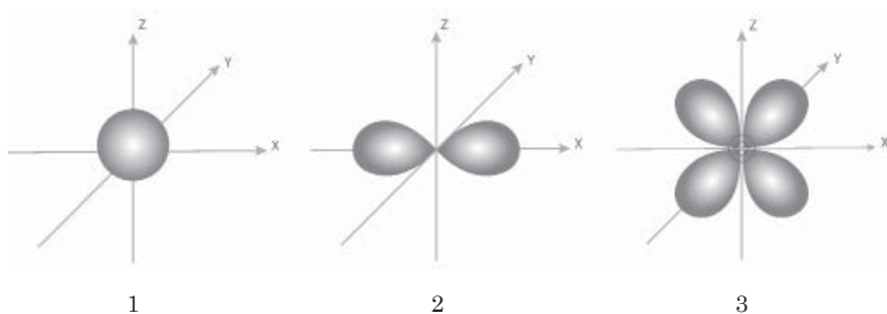
Obrázek č. 3. Různé tvary elektronového oblaku („geometrie“ kvantové chemie)
