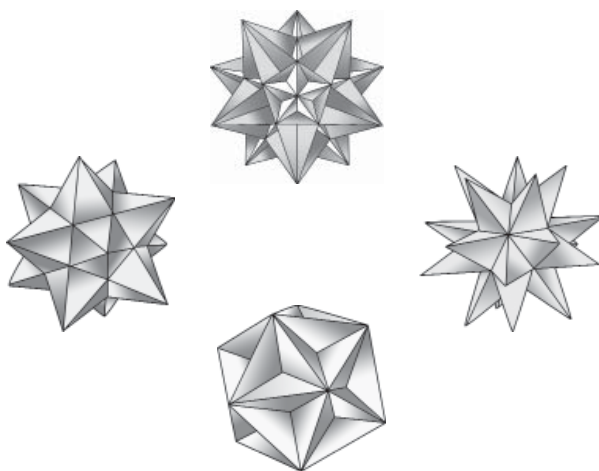
Obrázek č.62. Hvězdicové mnohostěny: Kepler-Poinsotová tělesa
