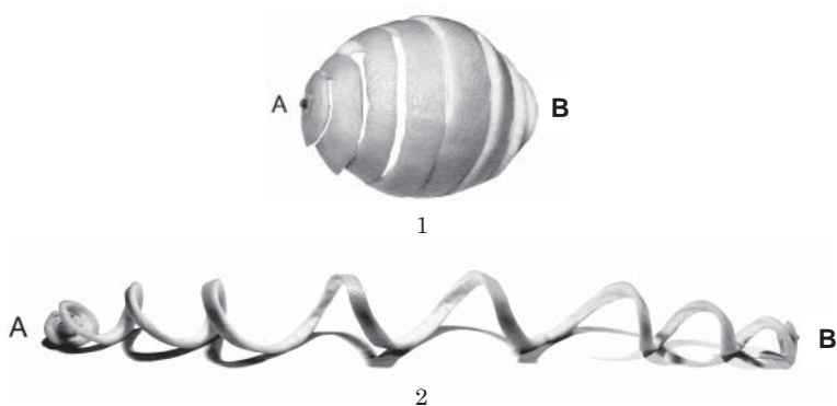
Obrázek č. 4. Názorný příklad přeměny elektronu z částice na vlnu:
