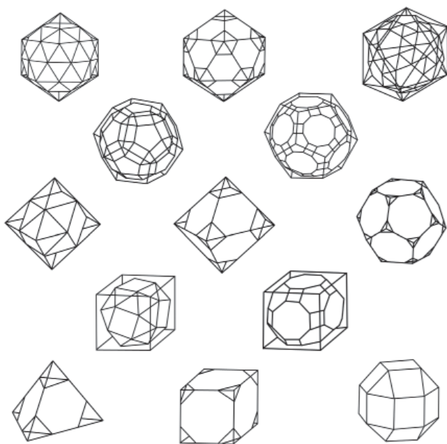
Obrázek č. 60. Prapůvodní schéma rozmístění 13 poloprávdelných mnohostěňů
