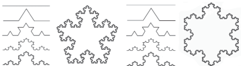
Obrázek č. 66. Fraktál Sněhová vločka Kocha
